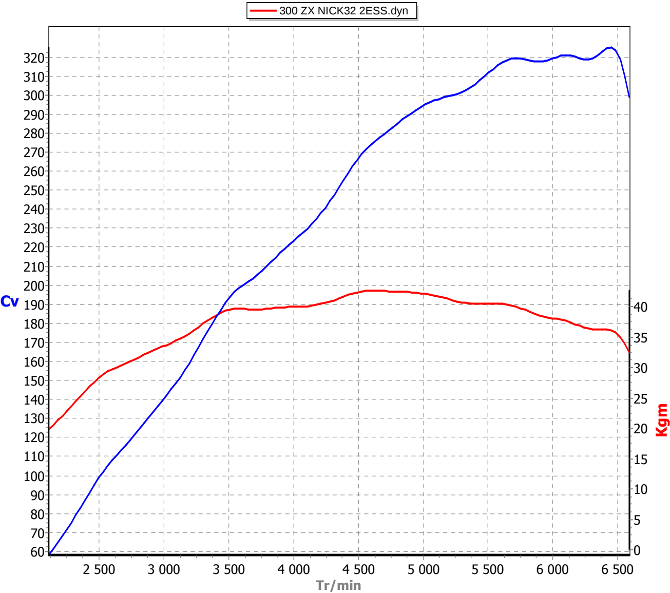
Couple/Puissance moteur
